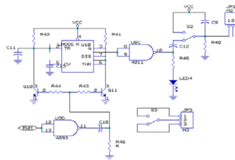
Figura 14. Circuito de Vigilancia
