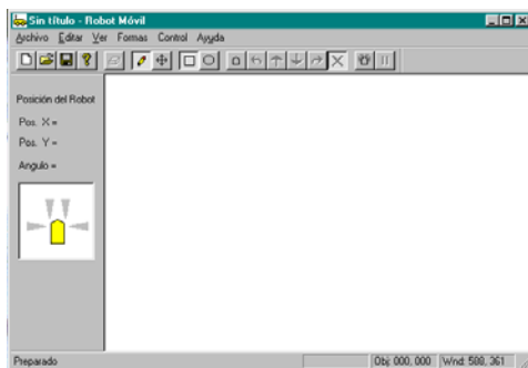
Figura 3 Interfaz Gráfica
