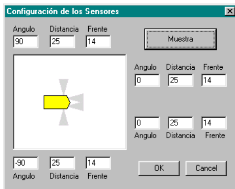
Figura 7 Configuración de Sensores
