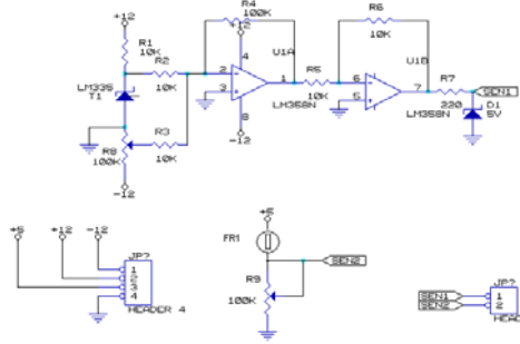
Figura 12. Sensores de Temperatura y Luz
