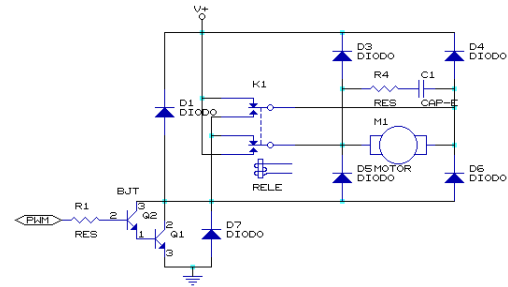
Figura 13. Control de Velocidad de Motores DC
